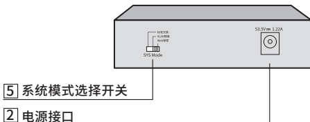
图1-14 TL-SG2005P后面板示意图
