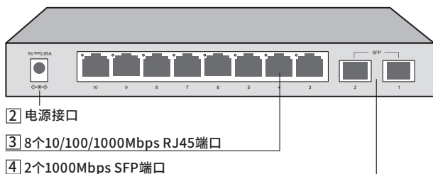
图1-4 TL-SG2210后面板示意图
