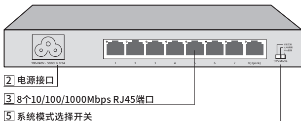
图1-6 TL-SG2008后面板示意图
