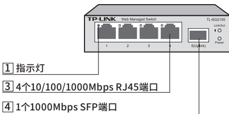
图1-8 TL-SG2105前面板示意图
