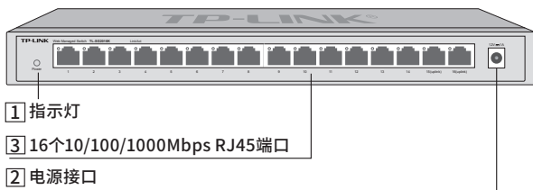
图1-1 TL-SG2016K前面板示意图
