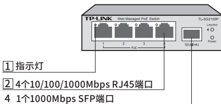
图1-13 TL-SG2105P前面板示意图
